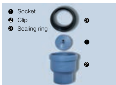
POLO-KAL NG condensate discharge element (FIGURE 43)
